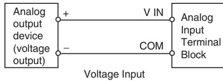
CP1E-NA20DR-A
